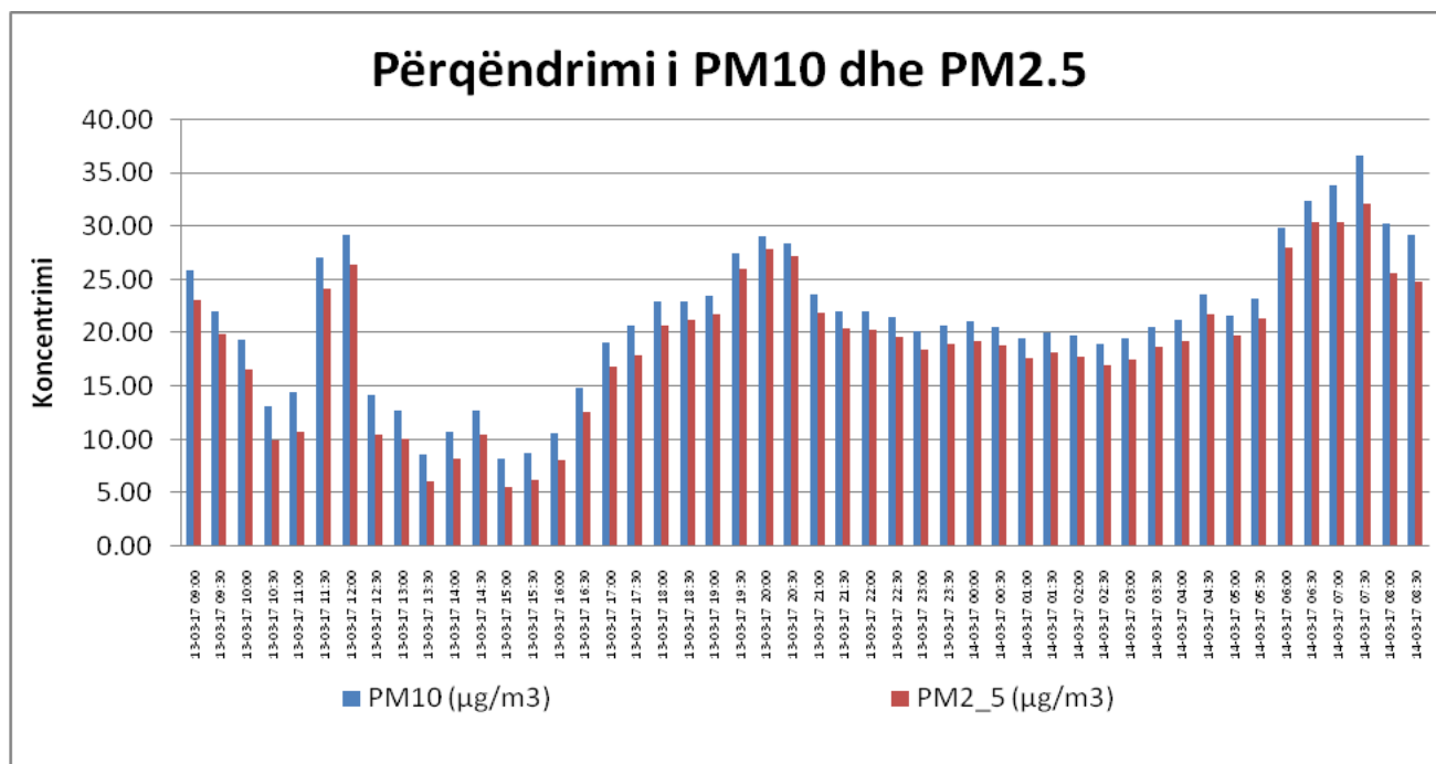
Fig. Nr.1 Paraqet përqëndrimin e PM10 dhe PM2.5 në Prishtinë
